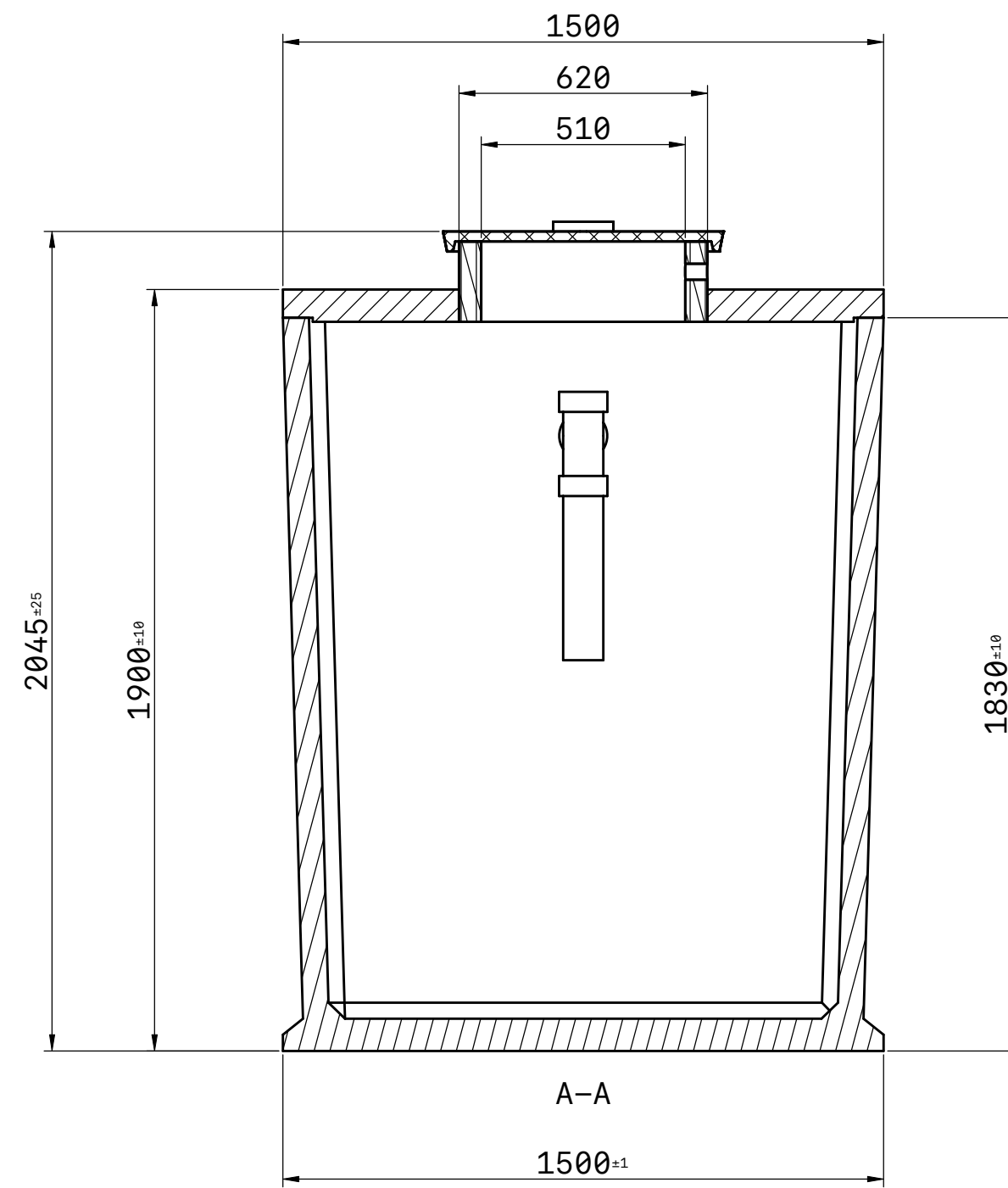
500mm ID Manhole Lid & Riser
